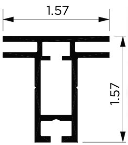
40mm SEG EXTRUSION
