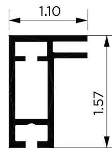
30mm SEG EXTRUSION
